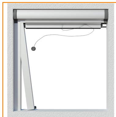
5. Inserire le guide spazzolino SX e DX all'interno delle guide registrabili con le alette dei ganci guida rivolte verso l'esterno (vedi particolare 2). In presenza di fuori squadra, effettuare le operazioni di registrazione delle guide spazzolino
