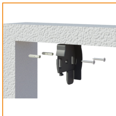
1. Fissare le testate a muro SX e DX
