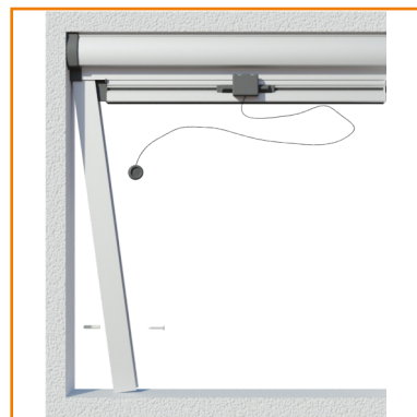
4. Inserire le guide registrabili SX e DX all'interno della feritoia del cassonetto e nell'invito testata a muro (vedi particolare 1). Fissare al vano
